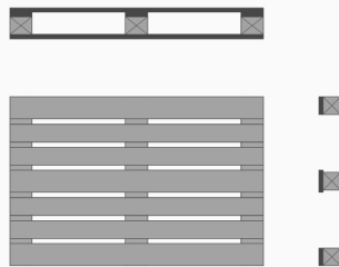
CP5 760 × 1140 mm
