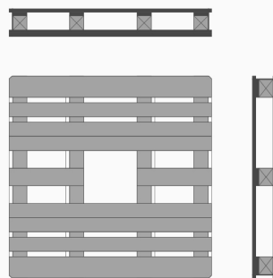
CP8 1140 × 1140 mm
