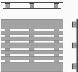
CP4 1100 × 1300 mm
