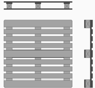
CP3 1140 × 1140 mm
