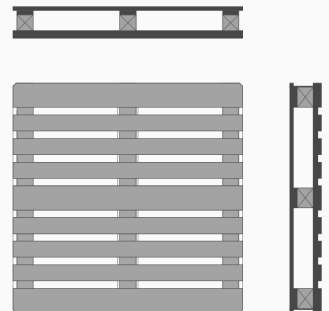
CP9 1140 × 1140 mm
